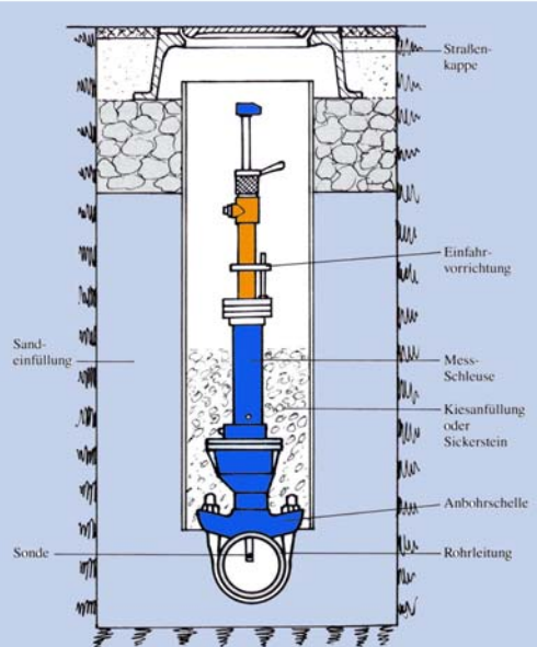
Mess - Punkt im Unterflureinbau
