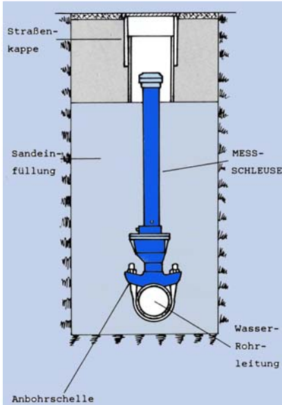
Mess - Schleuse im Unterflureinbau
